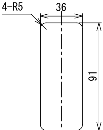
家具加工穴寸法
