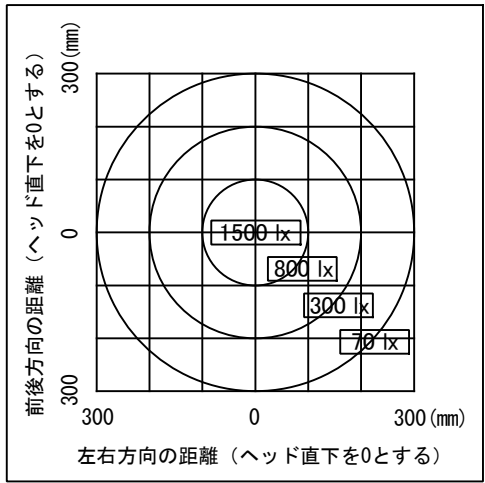
照度分布図
